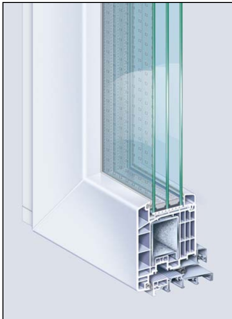
Das neue „Kömmerling 88plus“ Haustürsystem mit außen öffnendem Flügel.
