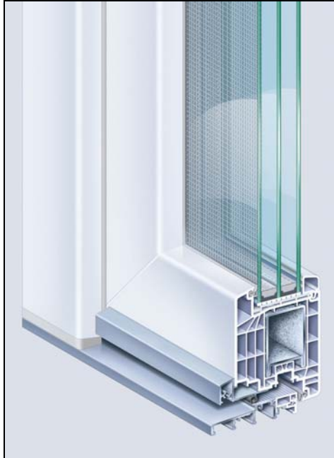
Das neue „Kömmerling 88plus“ Haustürsystem mit innen öffnendem Flügel.
