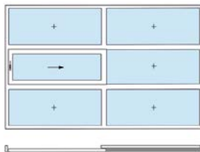
Двухстворчатая конструкция с глухой верхней и нижней фрамугой
